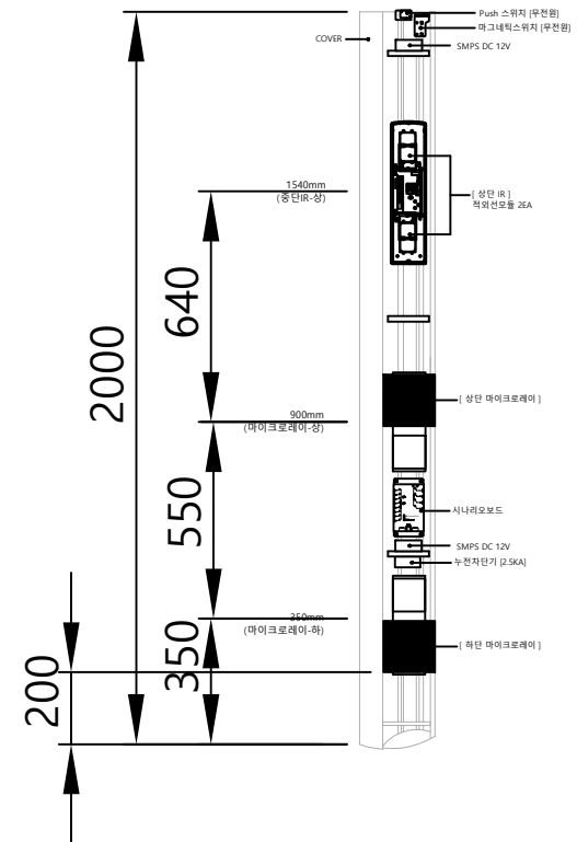
시스템 배치도
