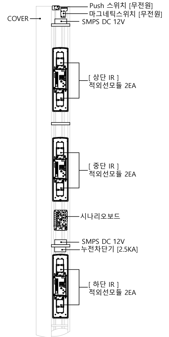
시스템 배치도
