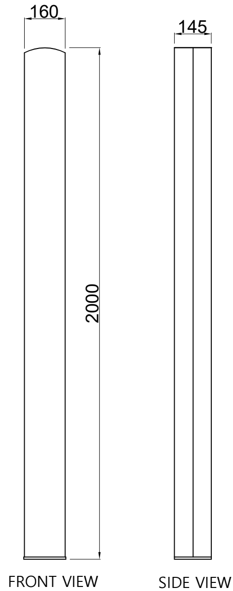
기기 외형도
