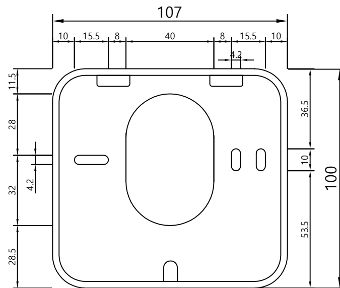
설치용 베이스
